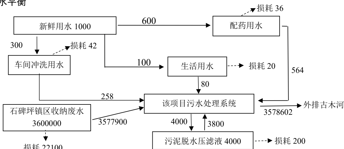
图2-1 该项目水平衡图（t/a）
